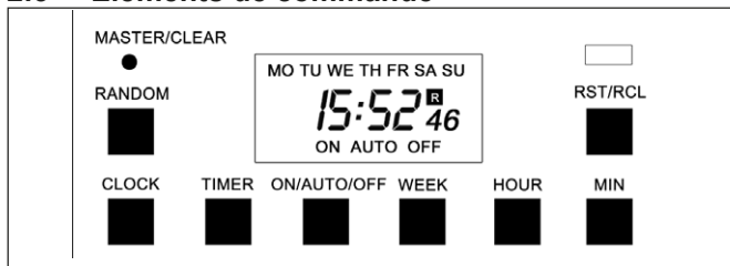
Fig.3: Éléments de commande
